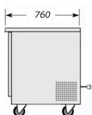
RIGHT ELEVATION
