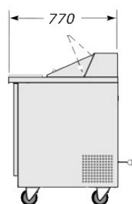
RIGHT ELEVATION
